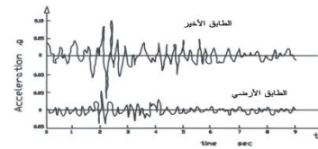
شكل (20-1): أكسيليو غرام زلزال سان فرانسيسكو (22.03.1957) في الاتجاه N-S للطابق الأرضي والطابق الأخير
