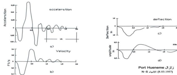
شكل (18-1): أكسيليو غرام هزات أرضية
