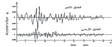
شكل (20-1): أكسيليو غرام زلزال سان فرانسيسكو (22.03.1957) في الاتجاه N-S للطابق الأرضي والطابق الأخير
